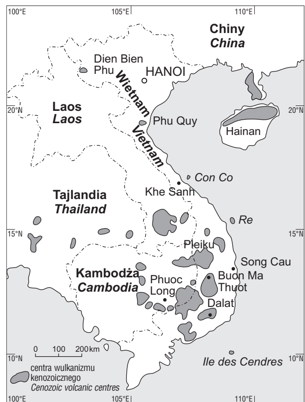
Ryc. 1. Centra kenozoicznego wulkanizmu bazaltowego w Azji SE (wg: Hoang i in., 1996a; Lee i in., 1998; uproszczone) Fig. 1. Cenozoic basaltic volcanic centres in SE Asia (based on Hoang et al., 1996 a; Lee et al., 1998; simplified)
