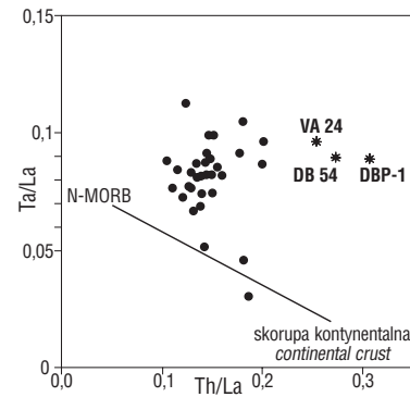
Ryc. 11. Diagram Ta/La w stosunku do Th/La dla bazaltów z Dien Bien Phu, w porównaniu z danymi dla pozostałych kenozoicznych bazaltów z Wietnamu (cytowanymi przez Hoanga i in., 1996a)
