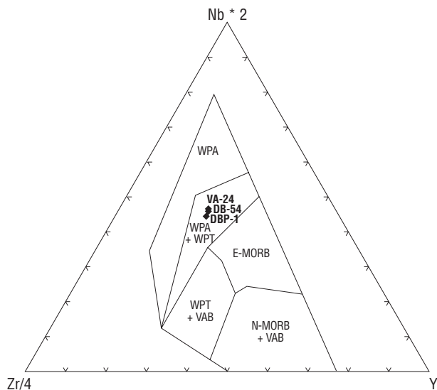
Ryc. 9. Pozycja bazaltów z Dien Bien Phu na diagramie Zr/4–2Nb–Y (Meschede, 1986). Objasnienia pól: WPA–śródpłytowe bazalty alkaliczne, WPT–śródpłytowe toleity, VAB–bazalty łuków wyspowych, E–MORB–bazalty typu E–MORB, N–MORB–bazalty typu N–MORB
