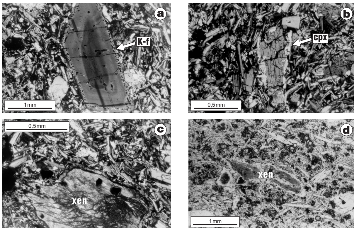
Ryc. 4. Wybrane przykłady minerałów zidentyfikowanych w próbkach DB 54 oraz VA 24; a — delikatne obwódki skaleni potasowego wokół fenokryształu plagioklazu (próbka DB 54), nikole skrzyżowane, x 40; b — fenokryształ piroksenu: klinopiroksen obrastający ortopiroksen (próbka DB 54), nikole skrzyżowane, x 40; c — ksenolit termicznie przeobrażonych skał otaczających: włóknisty fibrolit drobnokrystalicznego syllimanitu/mullitu oraz małe izometryczne kryształy spinelu Mg–Fe (próbka DB 54), nikole skrzyżowane, x 90; d — ksenolit termicznie przeobrażonych skał otaczających złożony z syllimanitu/mullitu oraz spinelu Mg–Fe (próbka VA 24), światło spolaryzowane, x 90
