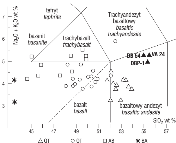
Ryc. 7. Pozycja bazaltów Dien Bien Phu na diagramie TAS (Le Maitre i in., 1989). Bazalty z Dien Bien Phu oznaczono trójkątami; pozostałe dane za: Hoang i in. (1996a) oraz Hoang & Flower (1998) Fig. 7. Plots of Dien Bien Phu basalts on the TAS diagram (Le Maitre i in., 1989). Dien Bien Phu basalts are marked by triangles; the other data taken from Hoang et al. (1996 a) and Hoang and Flower (1998)
