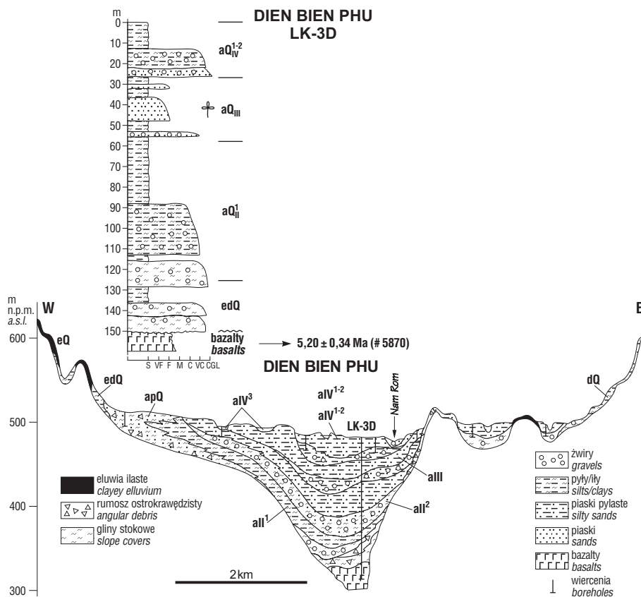
Ryc. 3. Profil i przekrój przez wiercenie LK-3D w mieście Dien Bien (wg danych N. D. Dy, inf. ustna 2002) wraz z lokalizacją próbki bazaltów datowanych metodą K-Ar; krzyżek na profilu litostratigraficznym oznacza znaleziska szczątków roślin
