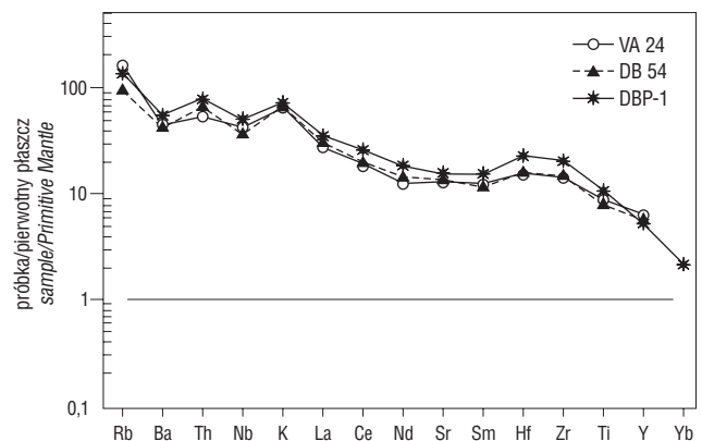
Ryc. 12. Diagram obrazujący rozkłady niedopasowanych pierwiastków w bazaltach z Dien Bien Phu, znormalizowanych względem pierwotnego płaszcz; DBP-1 — według Hoanga i in. (1996 a)
