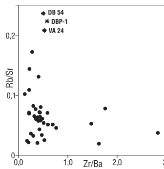
Ryc. 10. Diagram Rb/Sr w stosunku do Zr/Ba dla bazaltów z Dien Bien Phu, w porównaniu z danymi dla pozostałych kenozoicznych bazaltów z Wietnamu (cytowanymi przez Hoanga i in., 1996a)
