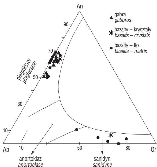
Ryc. 6. Pozycja skaleni z bazaltów Dien Bien Phu oraz zawartych w ksenolitach skał maficznych na diagramie Ab–An–Or (próbki DB 54, VA 24, LK-3D). Symbole oznaczają pochodzenie skaleni Fig. 6. Position of feldspars from Dien Bien Phu basalts and mafic xenoliths (samples: DB 54, VA 24, LK-3D) on the Ab–An–Or diagram. Symbols denote feldspar sources
