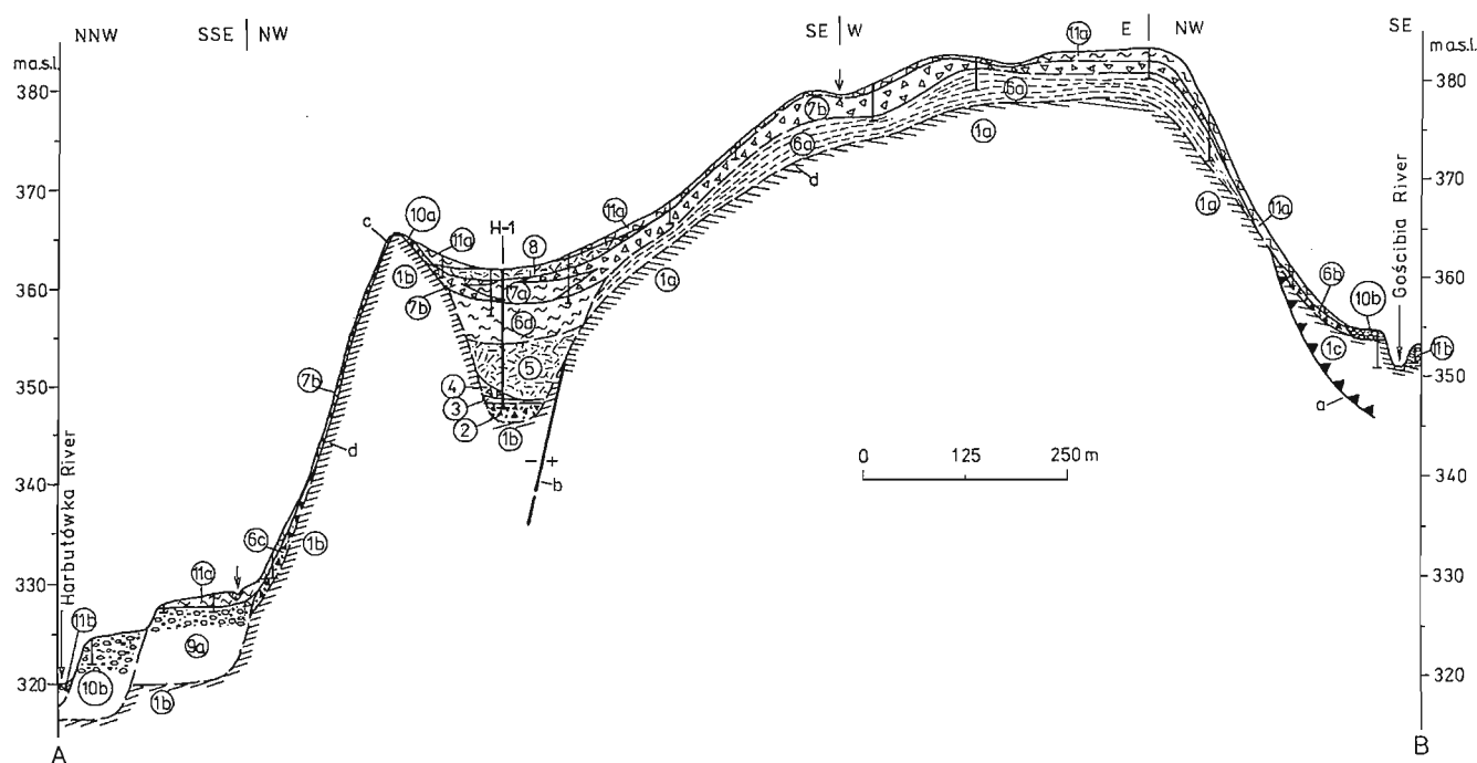
Fig. 3. Geologic cross-section A-B: flysch rocks according to M. Książkiewicz (1953) and M. Książkiewicz, J. Liszkowa (1979)
