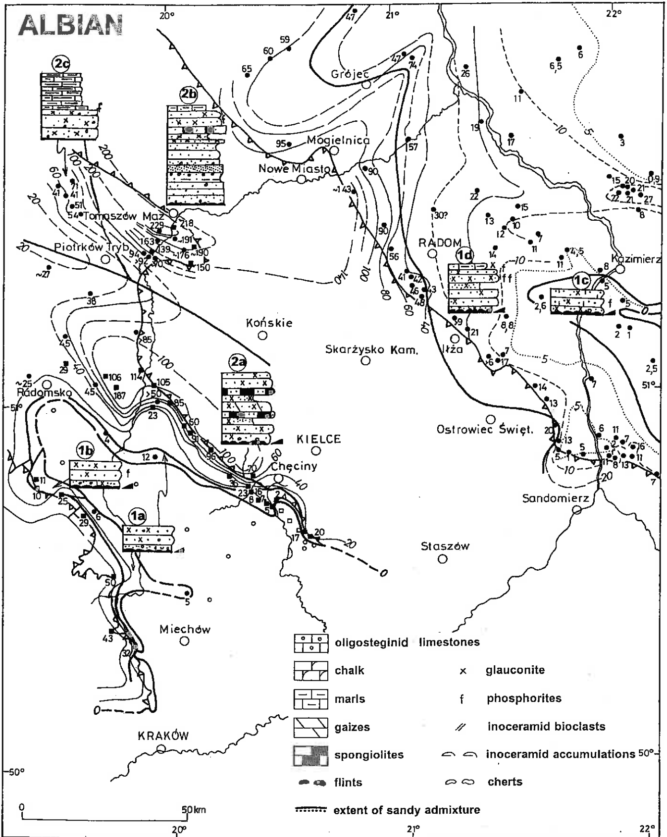
Fig. 4. Thickness and facies patterns of Albion deposits Explanations see Figs. 1 and 2 Rozkład miąższości i wykształcenie facjalne osadów albu Objaśnienia na fig. 1 i 2
