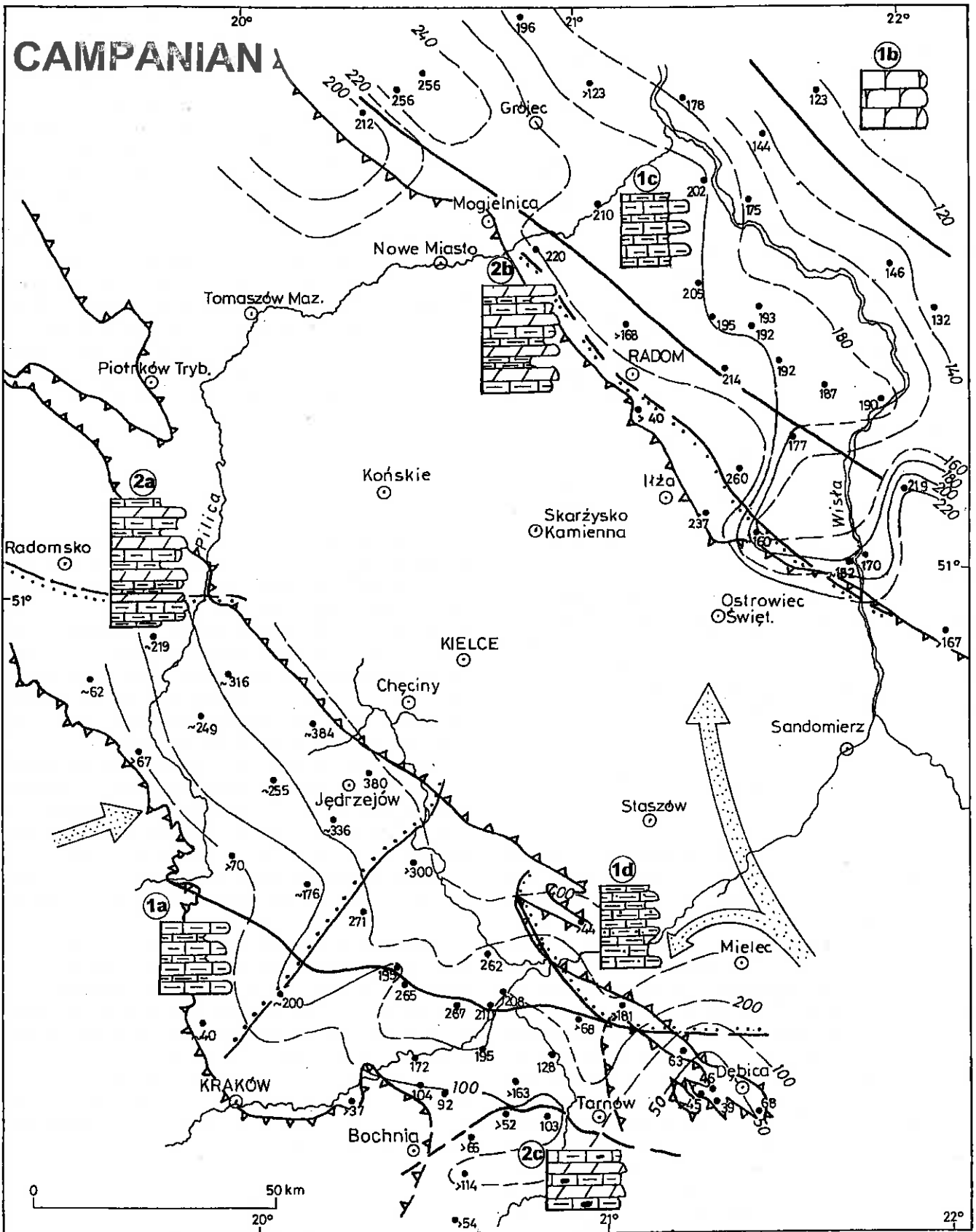
Fig. 9. Thickness and facies patterns of Campanian deposits Explanations see Figs. 1, 2 and 4 Rozkład miąższości i wykształcenie facjalne osadów kampanu Objasnienia na fig. 1, 2 i 4
