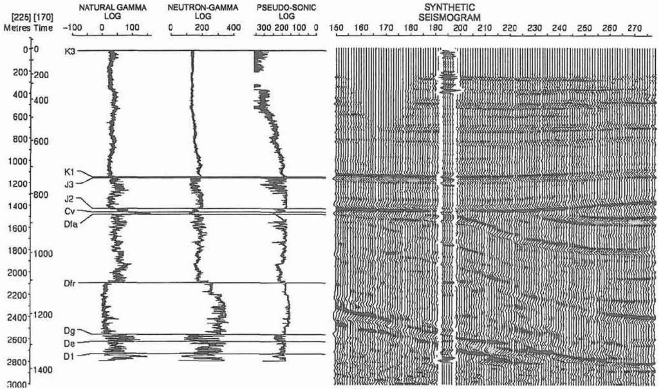
Fig. 3. Well Zakrzew IG 1 — natural gamma-ray log, sonic log, synthetic seismogram and its correlation with part of seismic line 24-5-80K Otwór Zakrzew IG 1 — krzywe karotazowe gamma i akustyczna, sejsmogram syntetyczny i jego korelacja z fragmentem linii sejsmicznej 24-5-80K
