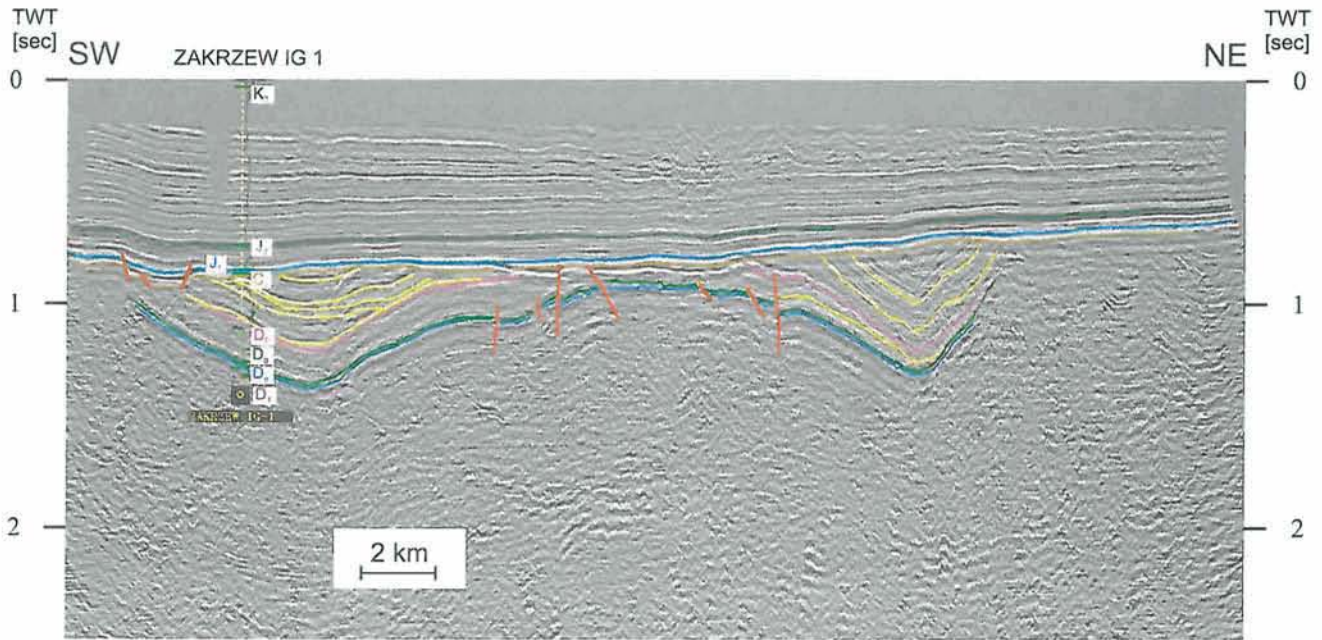
Fig. 4. Interpreted time seismic line 24-5-80K Interpretacja czasowego profilu sejsmicznego 24-5-80K
