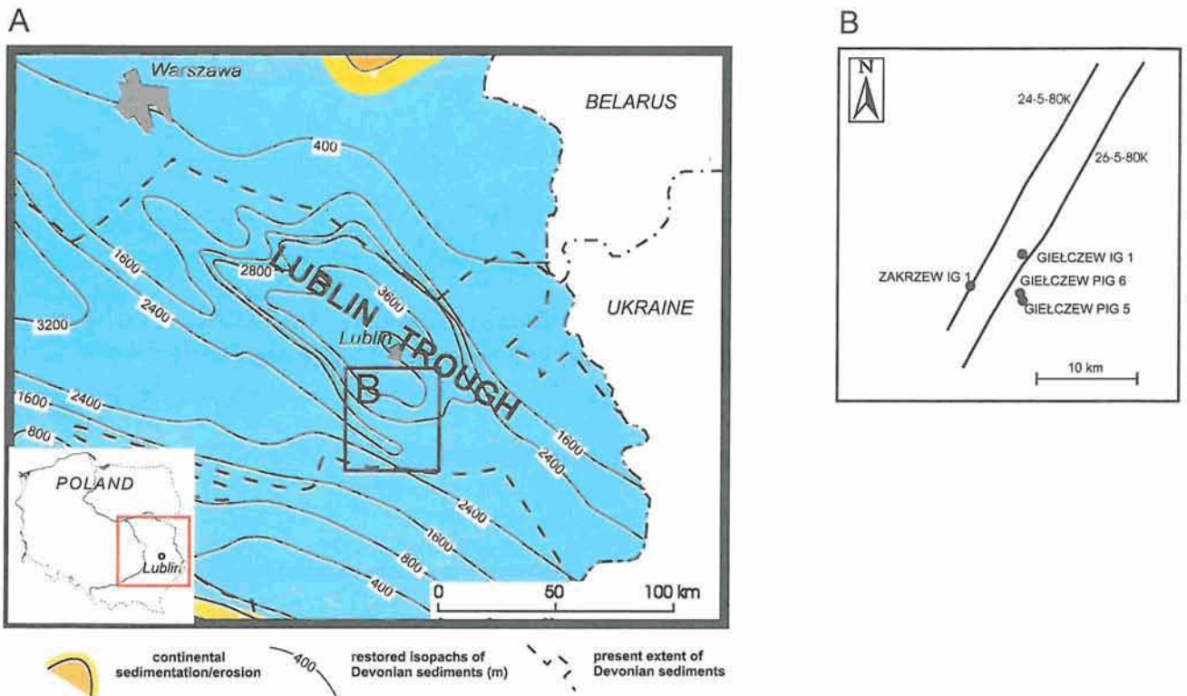
Fig. 1. A. Location map of the study area against the restored Devonian geometry of the Lublin Trough B. Location of investigated seismic lines and wells A. Lokalizacja obszaru badań na tle odtworzonej pierwotnej geometrii dewońskiego rowu lubelskiego B. Lokalizacja badanych linii sejsmicznych i wierceń
