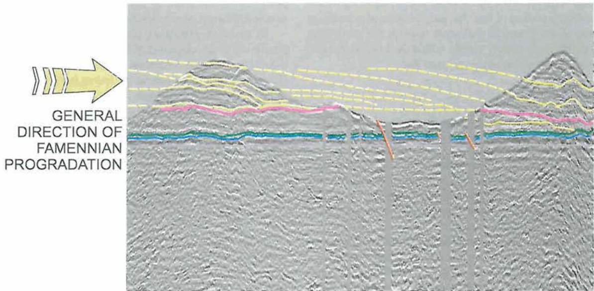
Fig. 7. Lower Famennian depositional model based on seismic line 24-5-80K Model depozycji famenu dolnego na podstawie profilu sejsmicznego 24-5-80K
