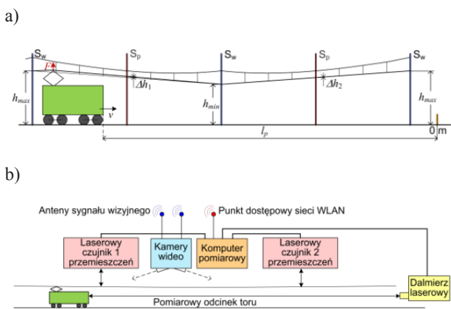
Rys. 3. Struktura i wyposażenie stanowiska pomiarowego: a) wyprofilowany odcinek sieci jezdnej, gdzie: $S_w$ – słupy wsporcze sieci, $S_p$ – słupy pomiarowe z zamontowanymi czujnikami pomiaru przemieszczenia przewodu wraz z osprzętem, $h_{max}$ – maksymalna wysokość robocza odbieraka, $h_{min}$ – minimalna wysokość robocza odbieraka; b) urządzenia pomiarowo-rejestrujące stanowiska
