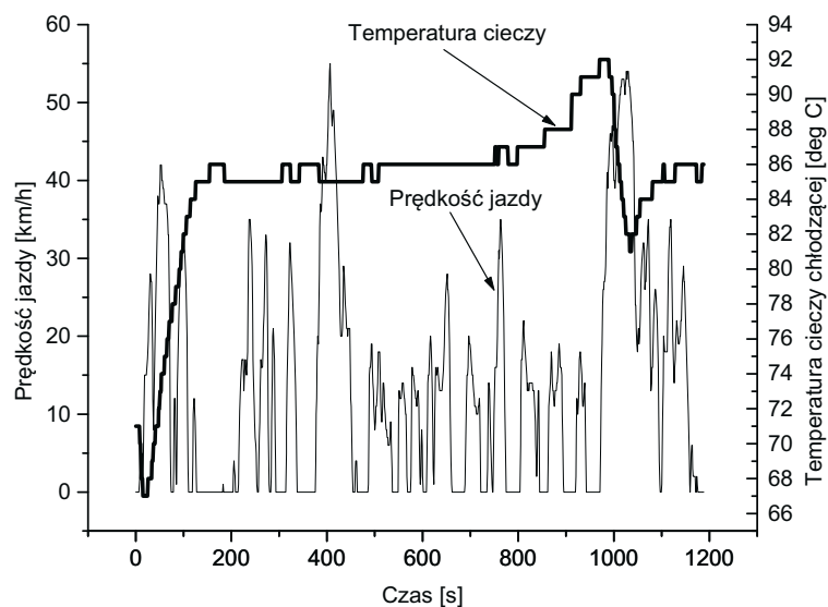
Rys. 7. Prędkość jazdy i temperatura cieczy opuszczającej głowicę podczas wybranej jazdy miejskiej w warunkach dużego natężenia ruchu Fig. 7. Car speed and coolant temperature during city road in traffic
