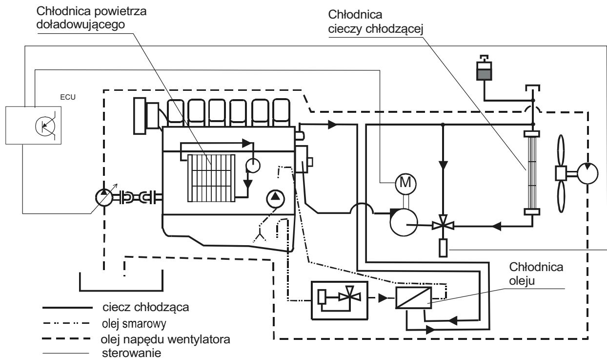
Rys. 10. Schemat układu chłodzenia silnika spalinowego lokomotywy Fig. 10. Cooling circuit for the rail engine
