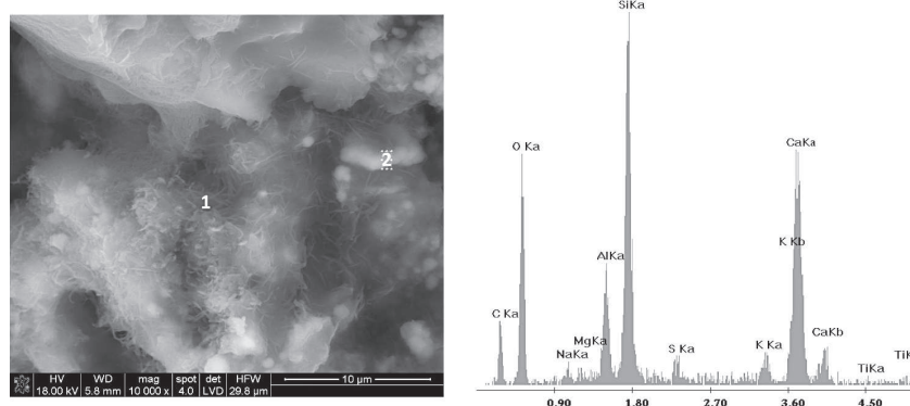
Ryc. 3. ABK z zastosowaniem CEM V/A (S-V) 32,5 R-LH – cementownia 4 z uwzględnieniem C/S – widoczny produkt C-S-H typu plaster pszczeli [1]
