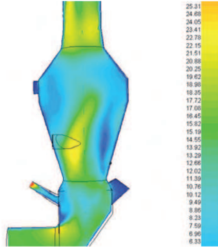
Źródło: Opracowanie własne. Ryc. 5. Rozkład prędkości
