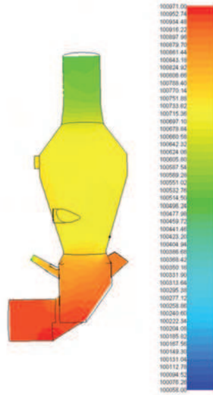
Źródło: Opracowanie własne. Ryc. 4. Rozkład ciśnienia
