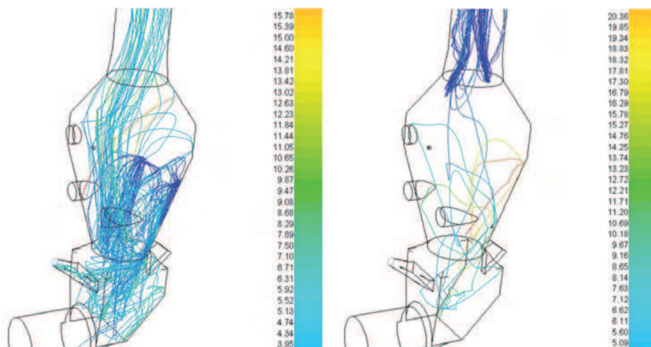
Ryc. 8. Wybrane trajektorie cząstek wszystkich frakcji z dolnego i górnego wyspu mąki
