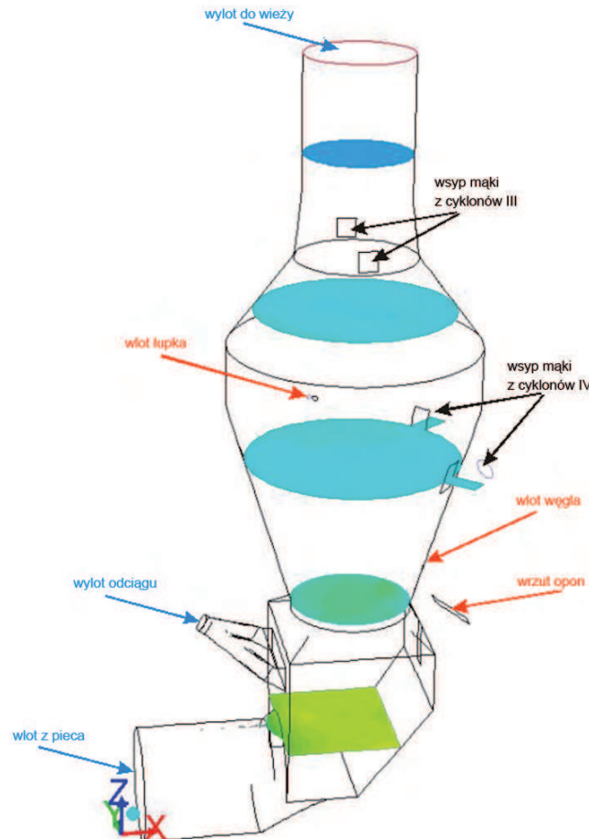
Ryc. 2. Geometria komory wzniosu i przekroje kontrolne
