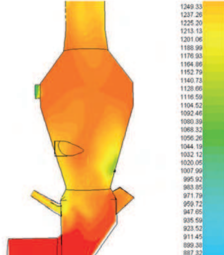
Źródło: Opracowanie własne. Ryc. 7. Rozkład temperatury
