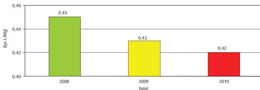
Ryc. 3. Zużycie paliwa na 1 Mg produkcji
