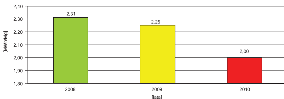
Rys. 2. Zużycie energii elektrycznej na 1 Mg produkcji
