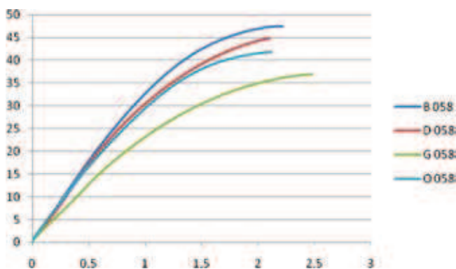
Rys. 2. Zależności \sigma-\epsilon przy doraźnym, jednoosiowym ściskaniu betonów o w/c = 0,58 z różnymi kruszywami (wartości naprężeń na osi Y w MPa, a odkształceń na osi X w ‰)
