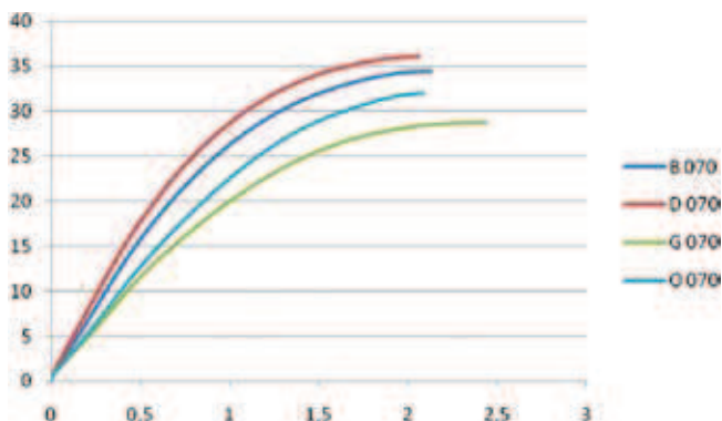
Rys. 1. Zależności \sigma-\epsilon przy doraźnym, jednoosiowym ściskaniu betonów o w/c = 0,70 z różnymi kruszywami (wartości naprężeń na osi Y w MPa, a odkształceń na osi X w ‰)
