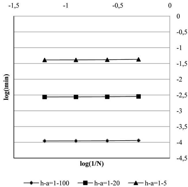
Fig. 20. Inf-sup test – cantilever plate h/a = 1/100, 1/20, 1/5 . S4R5 Abaqus element. Norm matrix S0 = M . Rys. 20. Test inf-sup – płyta wspornikowa h/a = 1/100, 1/20, 1/5 . Element Abaqus S4R5. Macierz normowa S0 = M
