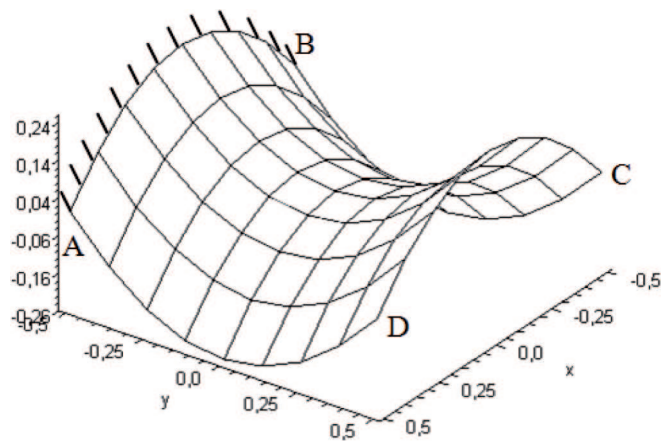
Fig. 1. Cantilever hyperbolic paraboloid. Rys. 1. Wspornikowa paraboloida hiperboliczna
