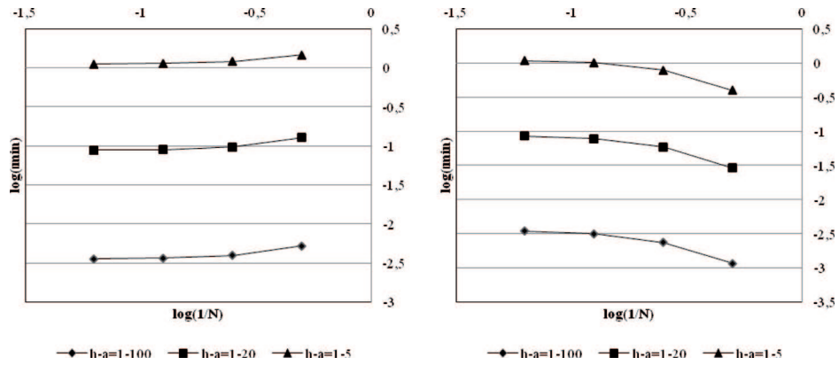
Fig. 19. Inf-sup test – simply supported plate h/a = 1/100, 1/20, 1/5 . Plate element with linear shape functions and uniformly reduced integration. Norm matrices S0 = M (left) and S01 (right). Rys. 19. Test inf-sup – płyta swobodnie podparta h/a = 1/100, 1/20, 1/5 . Element płytowy o liniowych funkcjach kształtu i całkowaniu zredukowanym. Macierze normowe S0 = M (po lewej) i S01 (po prawej)
