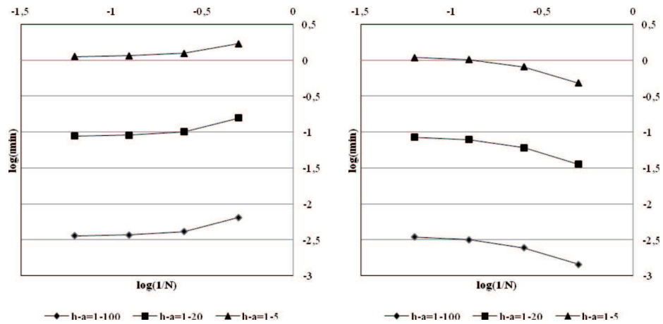
Fig. 16. Inf-sup test – simply supported plate h/a = 1/100, 1/20, 1/5 . Plate element with linear shape functions and selective/reduced integration. Norm matrices S_0 = M (left) and S_{01} (right). Rys. 16. Test inf-sup – płyta swobodnie podparta h/a = 1/100, 1/20, 1/5 . Element płytowy o liniowych funkcjach kształtu i całkowaniu selektywnie zredukowanym. Macierze normowe S_0 = M (po lewej) i S_{01} (po prawej)
