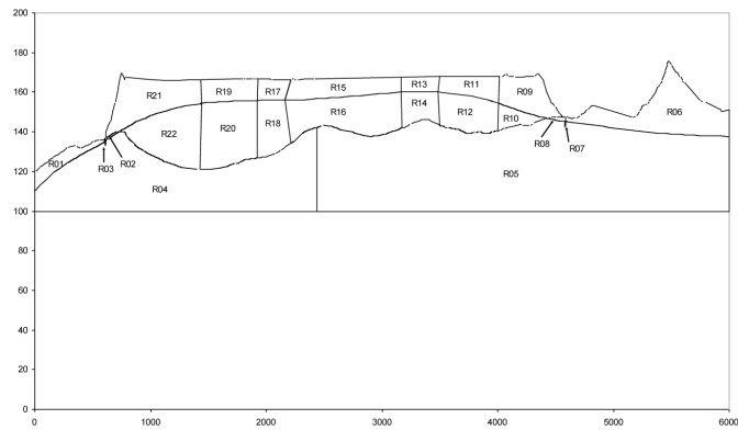
Fig. 6. Breakdown of the landfill area in the 2D regions. Rys. 6. Podział obszaru składowiska na regiony 2D
