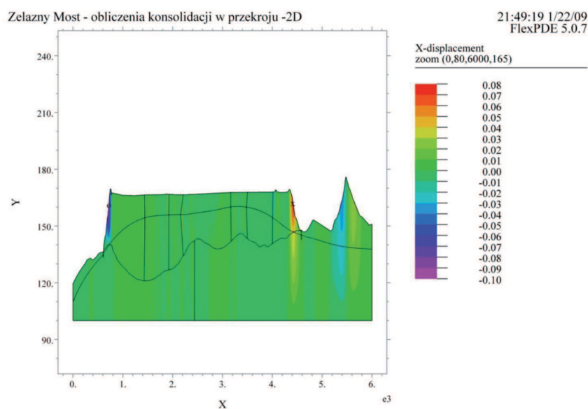
Fig. 8. Graph of horizontal displacement. Rys. 8. Wykres przemieszczeń poziomych
