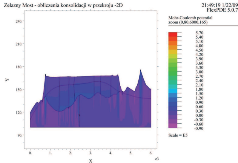
Fig. 12. Results for 2D model – Mohr-Coulomb potential. Rys. 12. Wykres potencjału Coulomba-Mohra
