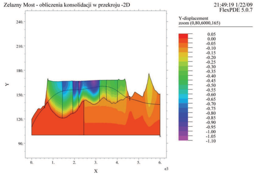
Fig. 9. Graph of the movements in the vertical direction. Rys. 9. Wykres przemieszczeń pionowych
