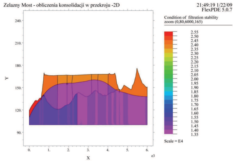
Fig. 10. Graph of \Phi potential. Rys. 10. Wykres potencjału \Phi
