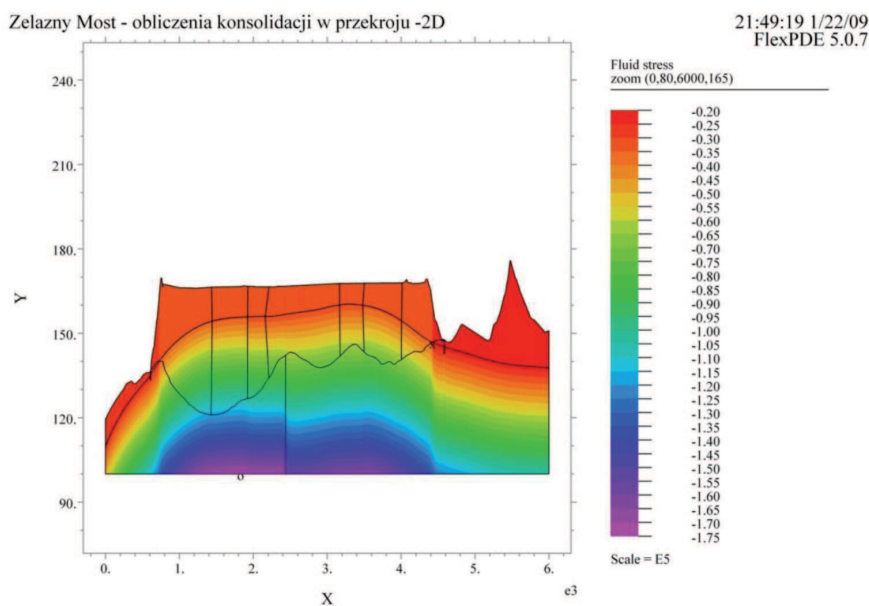
Fig. 11. Stresses in the liquid. Rys. 11. Wykres naprężeń \sigma w cieczy
