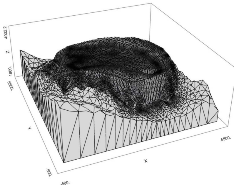
Fig. 2. View of spatial finite element mesh for the "Żelazny Most" landfill. Rys. 2. Widok przestrzennej siatki elementów skończonych dla zbiornika Żelazny Most
