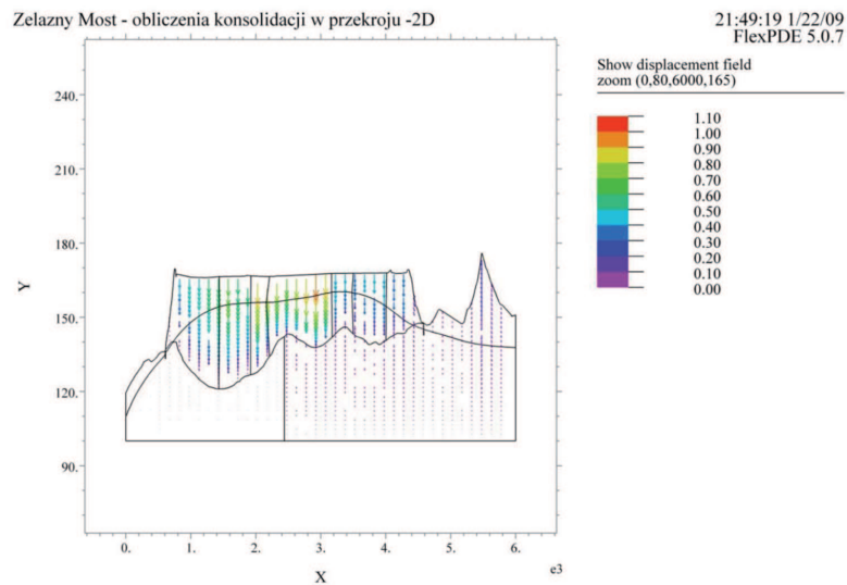
Fig. 7. Vector field of movements of material from the landfill. Rys. 7. Pole wektorowe przemieszczeń materiału składowiska
