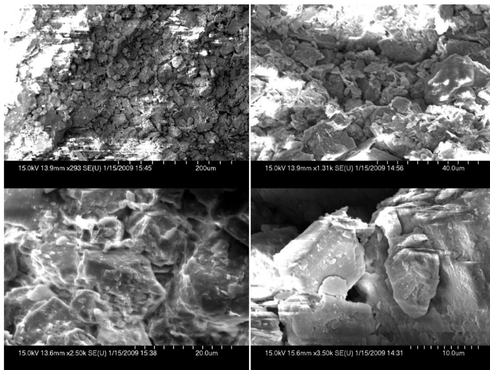
Fig. 5. Microscopic view of the test soil. Rys. 5. Widok mikroskopowy badanego gruntu
