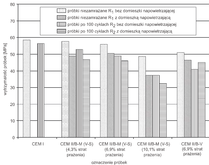
Ryc. 7. Mrozoodporność betonów
