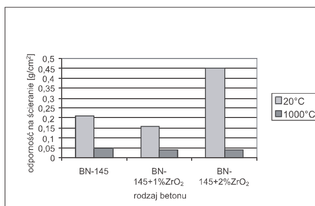
Ryc. 2. Ścieralność betonów ogniotrwiałych z dodatkiem ZrO 2
