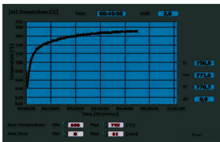
Ryc. 3. Przebieg badania niepalności zarejestrowany dla mieszanki gipsu budowlanego i mączki wapiennej w stosunku 1:1 z 0% dodatkiem składników organicznych
