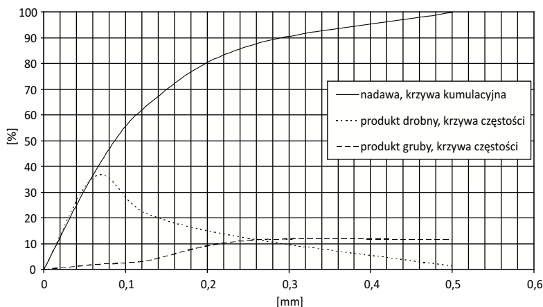
Ryc. 10. Wyznaczenie ziarna podziałowego dla produktów separatora cyrkulacyjnego
