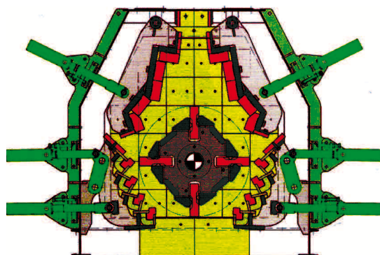
Ryc. 9. Przekrój kruszarki listwowej udarowej rewersyjnej firmy Hazemag [4]
