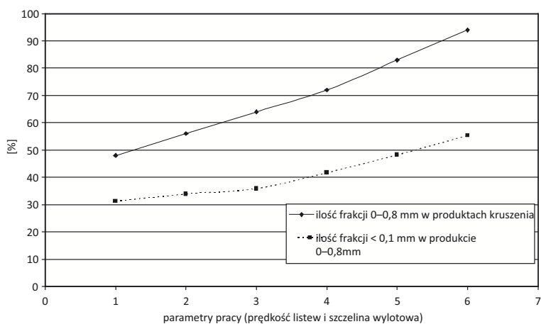
Ryc. 8. Przyrost ilości frakcji 0–0,8 mm i frakcji < 0,1 mm w produktach rozdrabniania w młynie młotkowym Hazemag
