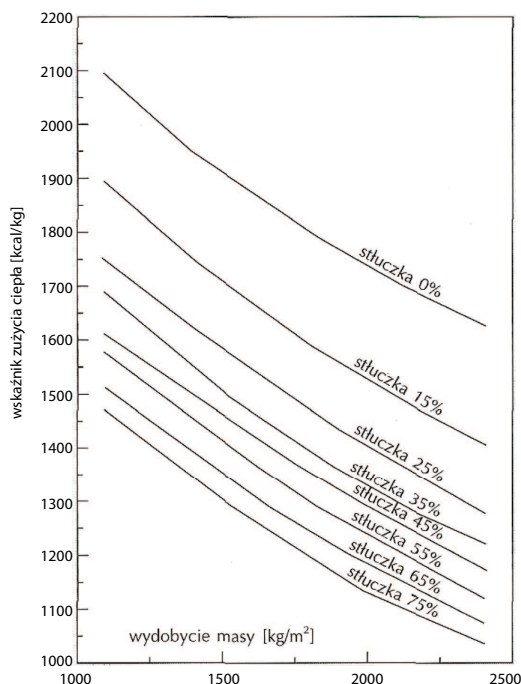
Ryc. 1. Wskaźnik zużycia ciepła dla pieca o powierzchni 100 m 2 w zależności od wydobywania masy szklanej i udziału stłuczki w zestawie [1]
