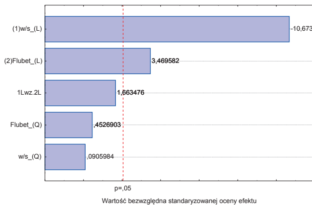
Wykres Pareto efektów standardyzow.; Wielkość: K lc S 2 wielk., 1 Bloki, 38 ukła; Czysty błąd MS=,0110636 ZZ K lc S
