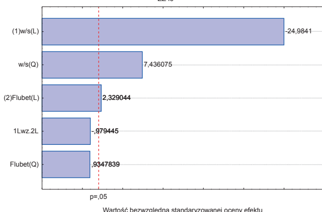
Wykres Pareto efektów standardyzow.; Wielkość: fc 2 wielk., 1 Bloki, 72 ukła; Resztowy MS = 7,126129 ZZ fc
