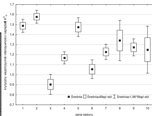
Rys. 4. Wyniki badań krytycznego współczynnika intensywności naprężeń K_{Ic}^S
