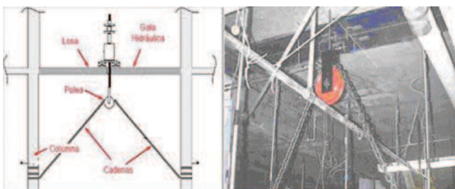
Rys. 3. Układy z ciągniami do realizacji obciążeń próbnych [12]
