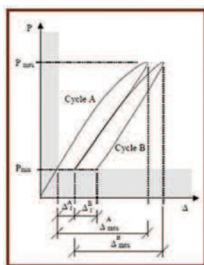
Rys. 5. Kryterium akceptacji – trwałość [12]
