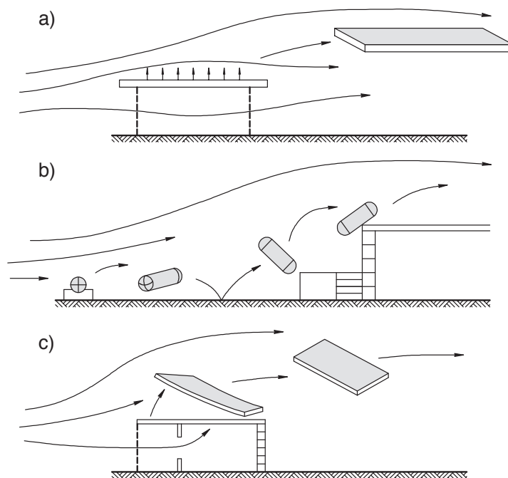
Rys. 5. „Pociski powietrzne” powstające w wyniku: a) sił aerodynamicznych, b) toczenia się i koziółkowania, c) ciśnienia wewnętrznego i zewnętrznego (rozerwania budynku) [8]
