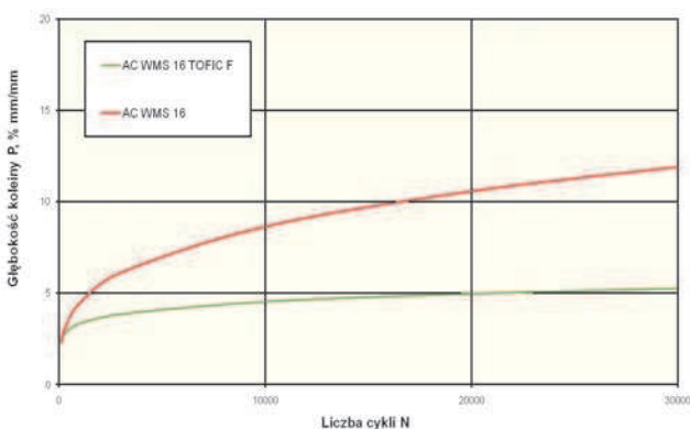
Rys. 6. Odporność na koleinowanie (duży aparat, 40°C) AC WMS 16 z dodatkiem włókna TOFIC® F
