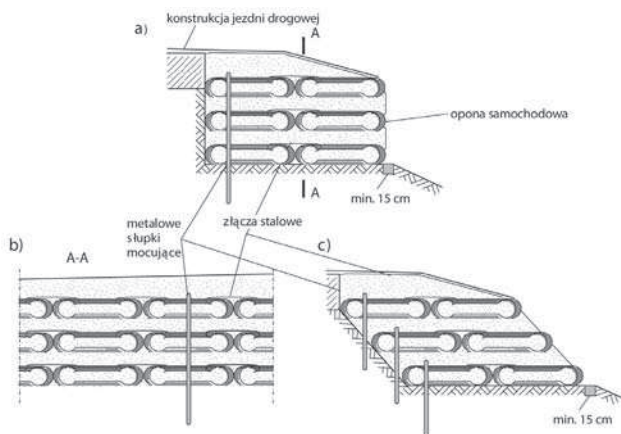
Rys. 4. Wzmocnienie poboczy drogowych zużytymi oponami
