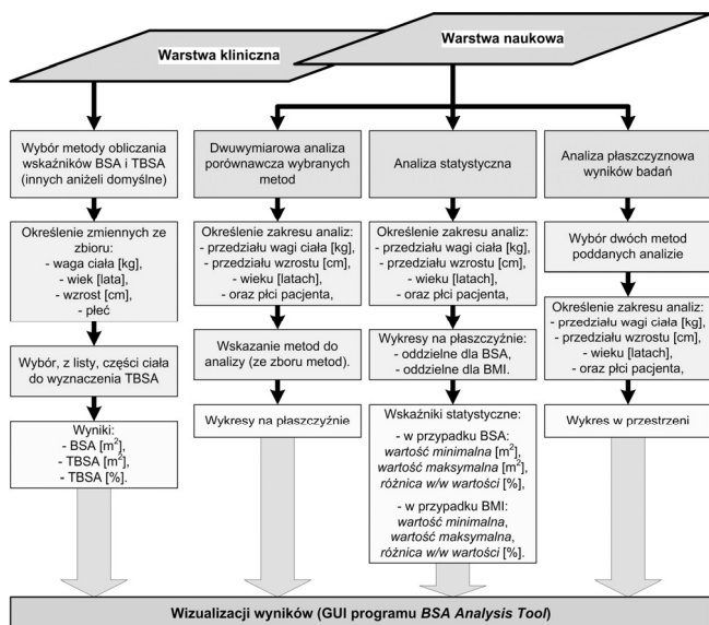
Rys. 1. Ogólna struktura opracowanego i wykonanego systemu BSA Analysis Tool Fig. 1. General structure of the developed BSA Analysis Tool system
