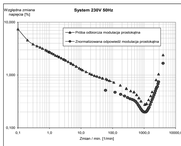
Rys. 1. Krzywa próby odbiorczej i znormalizowana odpowiedź flikermetra Fig. 1. Flickermeter performance test curve and normalized response
