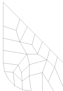
Fig. 1. Not optimized mesh for a partition plate of a hopper tank Rys. 1. Niezooptymalizowana siatka elementów skończonych dla przegrody zbiornika obłowego
