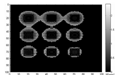
Rys. 6. Błąd bezwzględny rekonstrukcji głębokości umieszczenia defektów Fig. 6. Absolute error of the depth reconstruction of defect placement
