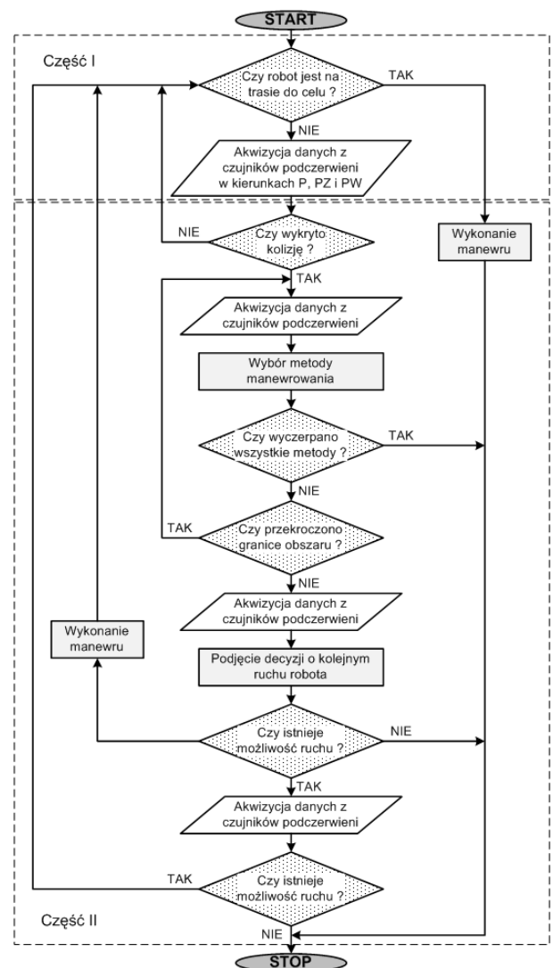
Rys. 3. Schemat algorytmu nawigacji bezkolizyjnej autonomicznego robota mobilnego SCORPIO
