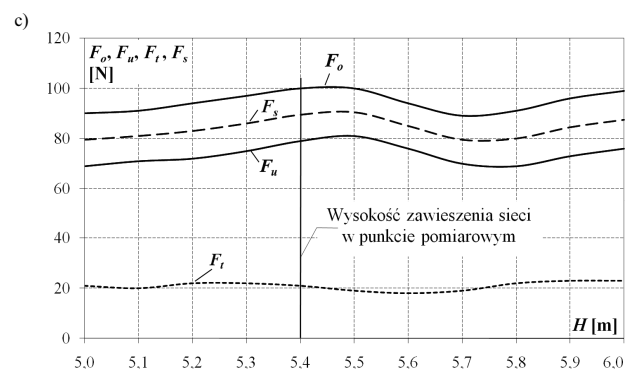
Rys. 7. Charakterystyki współpracy odbieraka z siecią: a) charakterystyki uniesienia przewodu jezdny w zależności od siły statycznej odbieraka i prędkości pojazdu; b) przebieg uniesienia przewodu dla wybranego odbieraka; c) charakterystyka statyczna siły nacisku przy obniżaniu F_o i unoszeniu F_u odbieraka, wartości siły średniej F_s oraz podwójnej siły tarcia F_t dla odbieraka z rys. b
