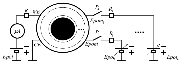
Rys. 3. Schemat układu pomiarowego
