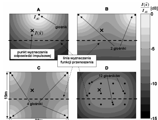
Rys. 1. Rozkład natężenia dźwięku w modelowym audytorium nagłaśnionym nieskorelowanymi falami generowanymi przez: A) pojedyncze źródło, B) dwa źródła, C) cztery źródła, D) 12 źródeł
