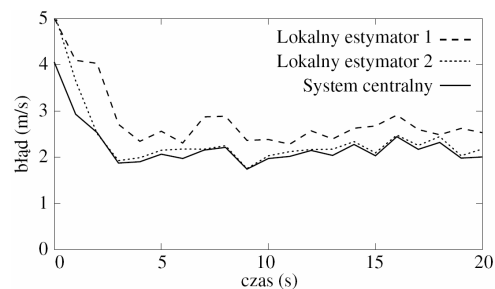
Rys. 5. Błędy wyznaczania prędkości w przypadku dużych zmian prędkości obserwowanego obiektu
