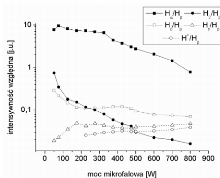
Rys. 4. Względne intensywności głównych linii emisyjnych w funkcji mocy mikrofalowej Fig. 4. Ratio of optical emission intensities of lines vs. microwave power
