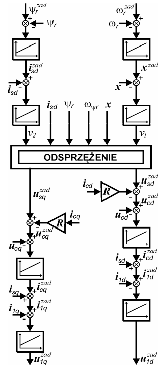
Rys. 3. Struktura układu nieliniowego, sterowania wektorowego silnika i filtra Fig. 3. Asynchronous motor and sinus filter nonlinear vector control system structure
