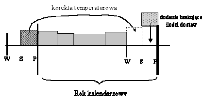
Rys. 6. Graficzna interpretacja korekt cyklu odczytu i różnicy warunków temperaturowych
