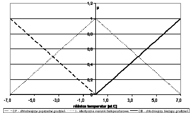
Rys. 7. Podział przestrzeni sygnału wejściowego różnica temperatur
