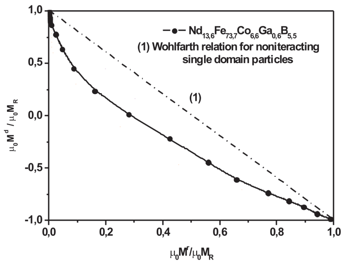
Fig. 1. Wohlfarth remanence curve for Nd 13,6 Fe 73,7 Co 6,6 Ga 0,6 B 5,5 magnet
