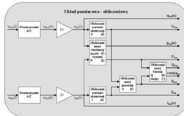
Rys. 3. Schemat blokowy układu pomiaru i obliczania parametrów instalacji elektrycznej
