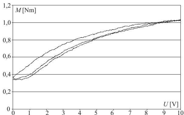
Rys. 9. Charakterystyka M=f(U) hamulca nr 3 Fig. 9. Brake's No. 3 characteristic M=f(U)
