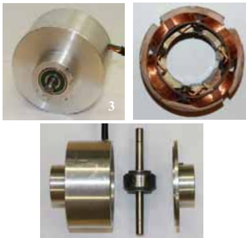
Rys. 8. Widok i budowa wewnętrzną hamulca wykonanego na bazie statora i wirnika silnika elektrycznego Fig. 8. View and internal structure brake made on the basis of electric motor's stator and rotor
