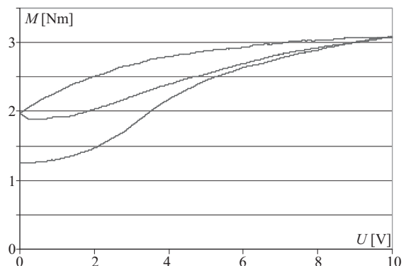
Rys. 7. Charakterystyka M=f(U) hamulca nr 2
