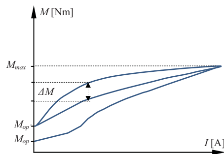
Rys. 10. Oznaczenia parametrów do obliczeń wielkości histerezy Fig. 10. Parameters to calculate the size of the hysteresis
