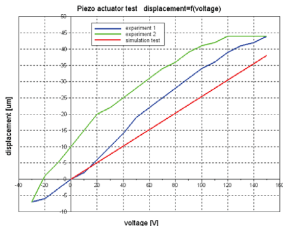
Fig. 11. Measurement results for piezostack actuator Rys. 11. Wyniki pomiaru przemieszczenia piezonapędu
