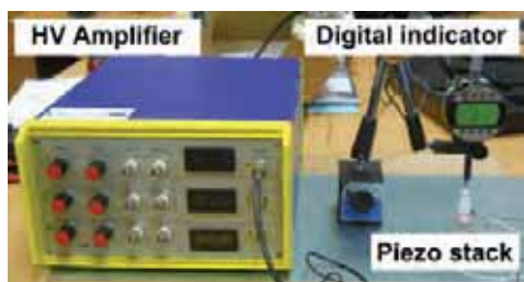
Fig. 10. Measurement arrangement for piezostack actuator Rys. 10. Stanowisko pomiarowe napędu piezoelektrycznego
