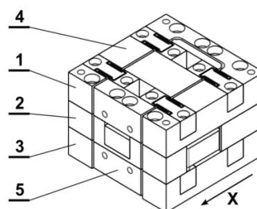
Fig. 1. A general concept of 1 DOF translational module Rys. 1. Moduł ruchu liniowego 1 DOF
