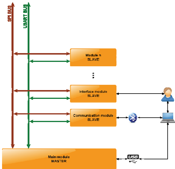
Fig. 3. Modules' organization scheme Rys. 3. Schemat organizacyjny modułów
