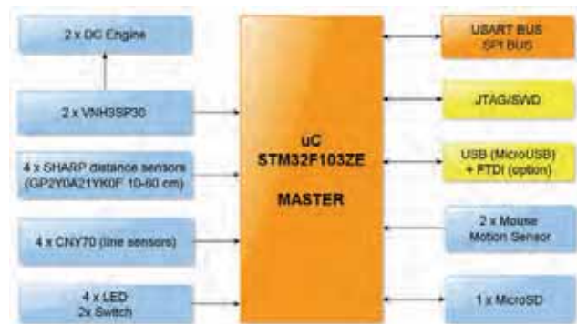
Fig. 4. Main module block diagram Rys. 4. Schemat blokowy modułu głównego
