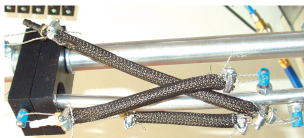
Fig. 9. Muscle system of the forearm Rys. 9. System mięśniowy przedramienia
