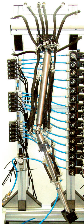
Fig. 6. Muscle system of the prototype Rys. 6. System mięśniowy prototypu
