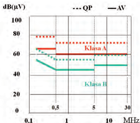
Rys. 1. Dopuszczalne poziomy emitowanych zaburzeń dla urządzeń klasy A i B dla przyłączy zasilania według PN-EN 55022 [4]
