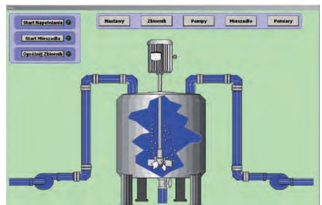
Rys. 7. Główne okno interfejsu operatora
