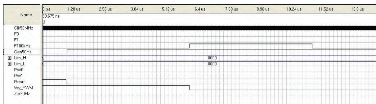
Rys. 4. Zerowanie modułu
