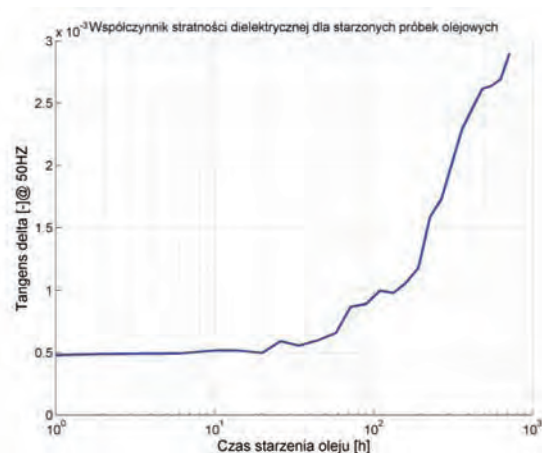
Rys. 3. Wykres zależności zmian współczynnika \text{tg}\delta od czasu starzenia próbek olejowych
