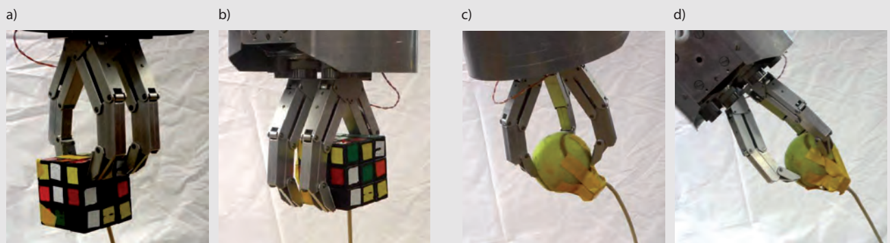
Rys. 6. Przykłady typowych zastosowań chwytaka wielopalczonego – chwytanie delikatnych obiektów o skomplikowanych kształtach Fig. 6. Typical applications of multifinger gripper – prehension of delicate objects with untypical shapes
