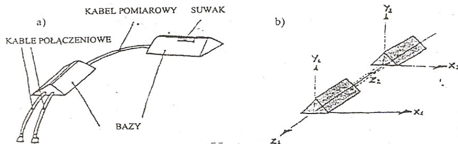
Rys. 7. Widok ogólny dwubiegunowego czujnika tensometrycznego firmy Biometrics Ltd. z Wielkiej Brytanii wraz z układem odniesienia
