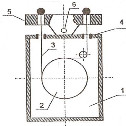
Rys. 6. Wzdłużny przekrój „mechanizmu turyńskiego”
