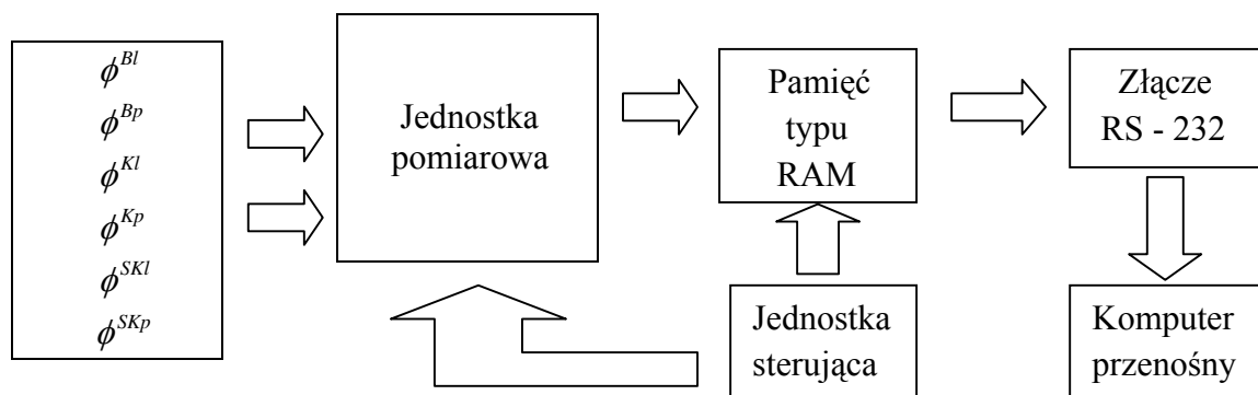
Rys. 9. Schemat blokowy cyfrowego układu rejestracji „surowych” kątów względnych osoby badanej, podczas chodu
