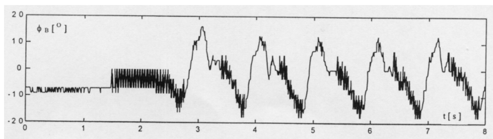
Rys. 10. Zarejestrowany przebieg „surowego” kąta względnego dla stawu biodrowego osoby badanej
