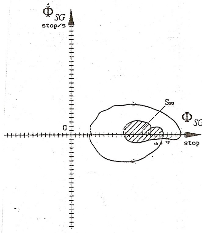
Rys. 4. Przykładowy wykres (typu \dot{\Phi}_{SG} = f_{1SG}(\Phi_{SG}) ) stawu skokowo-goleniowego zdrowego i sprawnego człowieka. Różnica t_k - t_p = T_- – jest to czas trwania fazy podporowej nogi z podłożem; S_{SG} – pole małej pętli. Wykres uzyskano w Centrum Bioinżynierii w Mediolanie, dla względnie stałej prędkości i częstotliwości kroczenia w płaszczyźnie strzałkowej ruchu po względnie płaskiej i utwardzonej powierzchni
