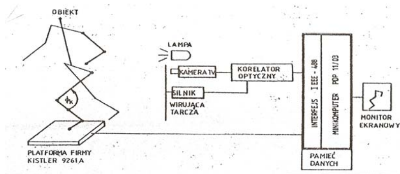
Rys. 5. System ELITE-3D z Centrum Bioinżynierii w Mediolanie, stosowany do rejestracji chodu i biegu człowieka [1]
