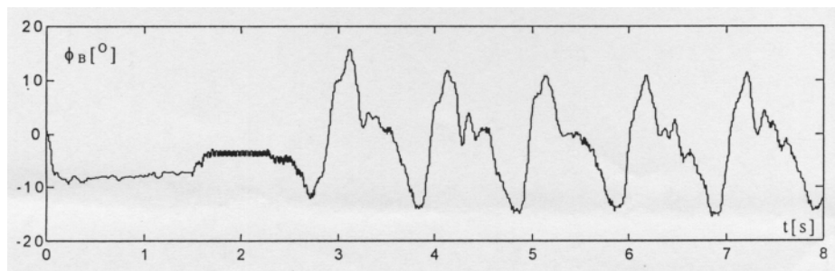
Rys. 11. Przebieg kąta względnego dla stawu biodrowego osoby badanej po zastosowaniu własnego cyfrowego filtra wielomianowego (w wersji programowej)
