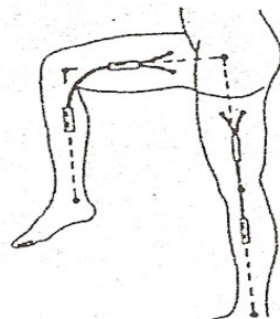
Rys. 8. Pomiar kąta względnego w stawie kolanowym człowieka za pomocą dwubiegunowego czujnika tensometrycznego firmy Biometrics Ltd.
