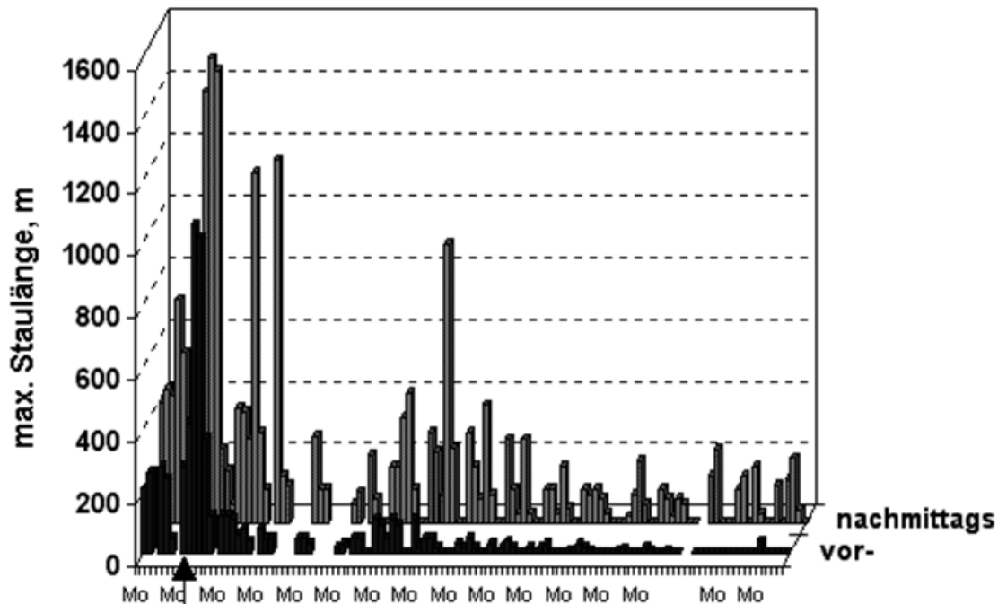
Fig. 4. Timeline of maximum morning (front) and afternoon (back) congestion lengths on Bismarck street, Heidelberg. Black triangle indicates time of reconstruction. Congestion lengths decrease exponentially Рис. 4. Время заторов максимальной длины на улице Бисмарка в Гейдельберге в утренние часы (спереди) и днем (сзади). Черный треугольник указывает время реконструкции. Длина затора убывает экспоненциально
