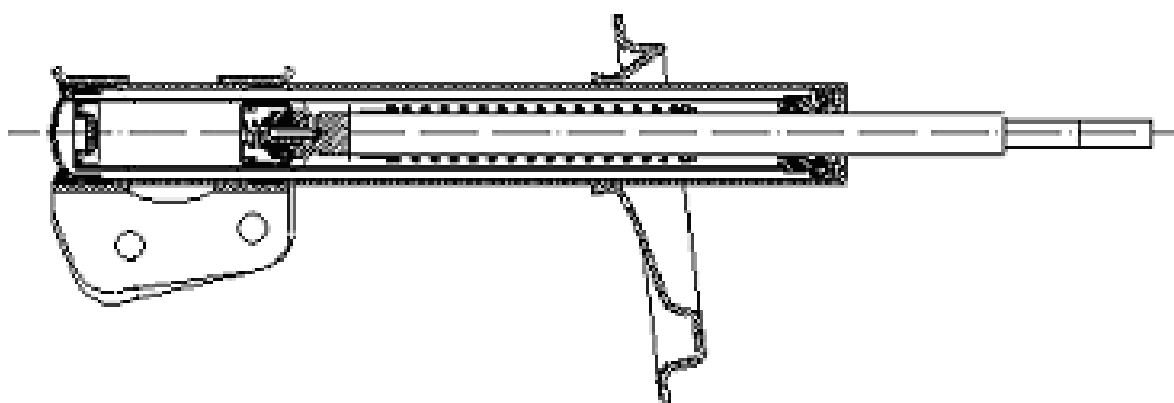
Fig. 3. Shock absorber construction Rys. 3. Budowa amortyzatora samochodowego
