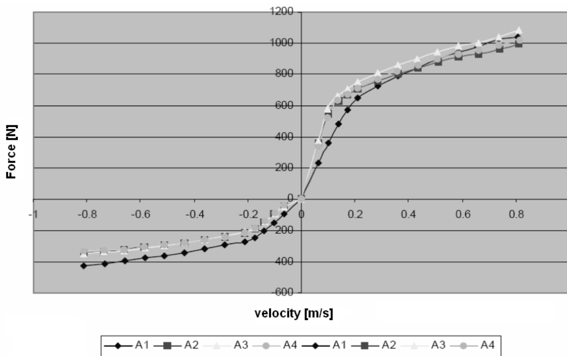
Fig. 2. Dumping characteristic of new schock absorbers Rys. 2. Charakterystyka tłumienia nowych amortyzatorów
