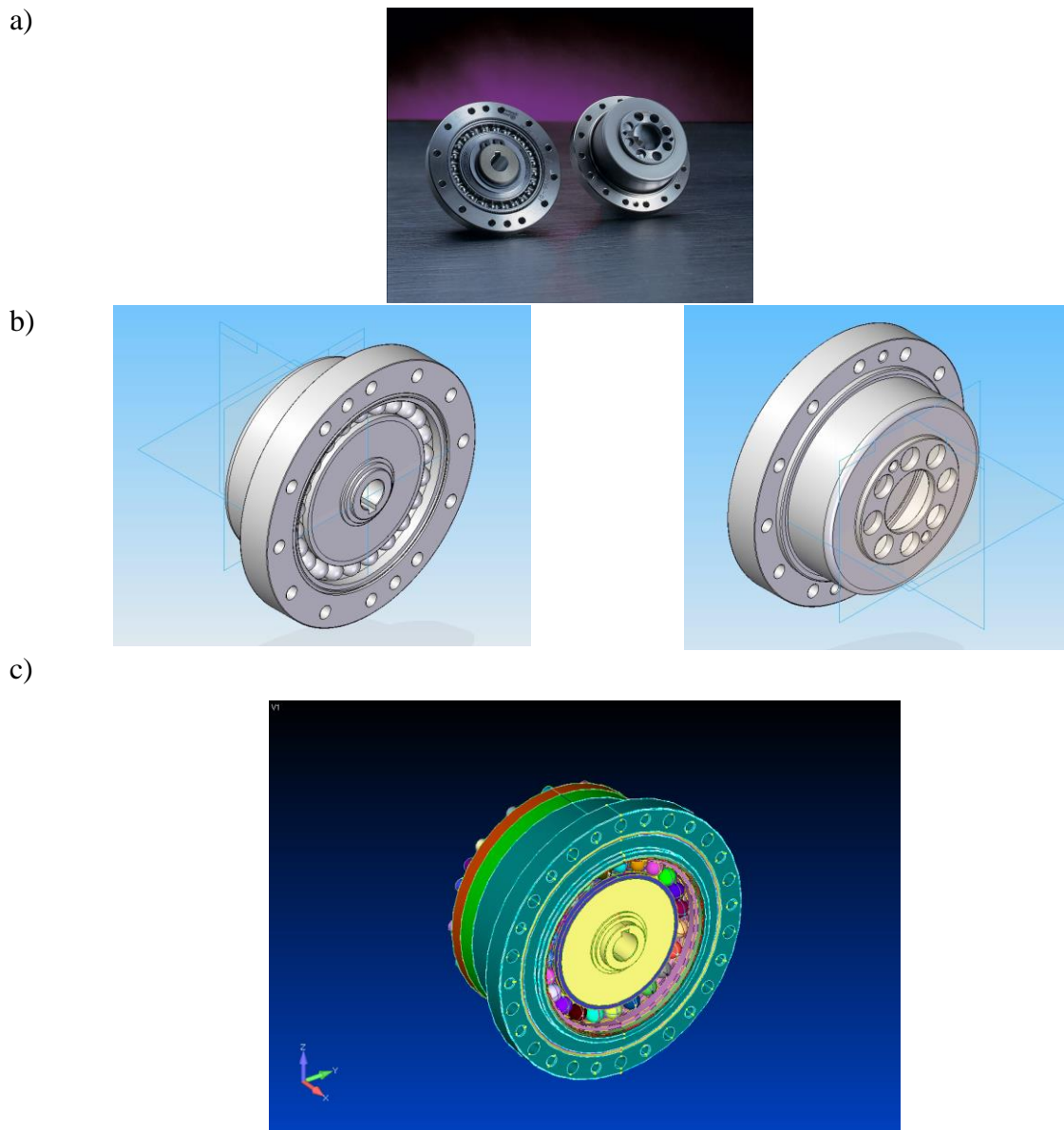
Rys. 1. a) Przekładnia falowa [2], b) model geometryczny przekładni, c) model numeryczny przekładni Fig. 1. a) Harmonic drive, b) geometric model of gear, c) numerical model of gear
