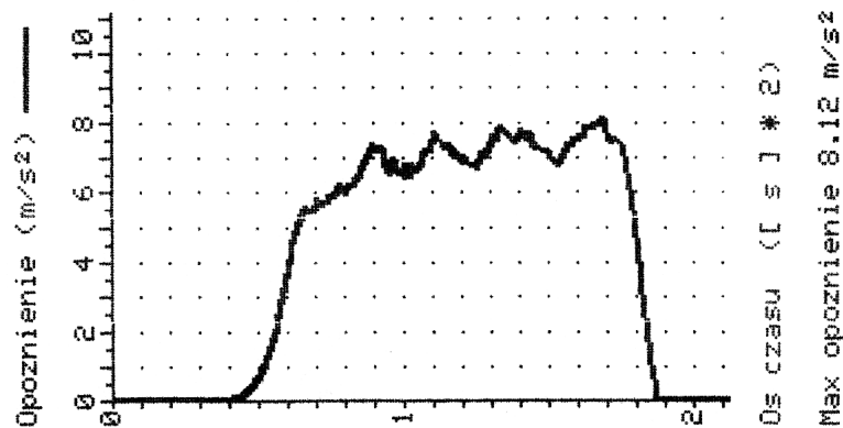
Fig. 4. Example of decelerometer printout Rys. 4. Przykład wydruku z opóźnieniomierza
