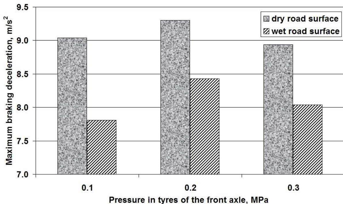
Fig. 5. Maximum deceleration in terms of type of surface and pressure in tyres of the front axle Rys.5. Maksymalne opóźnienie w zależności od rodzaju nawierzchni oraz ciśnienia powietrza w kołach przedniej osi
