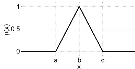
Fig. 5. A chosen input appurtenance function Rys. 5. Wybrana funkcja przynależności wejść
