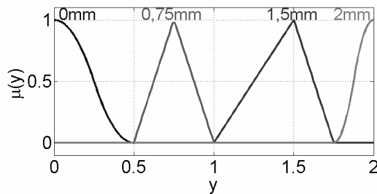
Fig. 7. Way number 1 of construction of the fuzzy outputs of the fuzzy logic system for a damage in the form of the chipping tip of the tooth Rys. 7. Sposób „1” budowy rozmytych wyjść systemu logiki rozmytej dla uszkodzenia w postaci wykruszenia wierzchołka zęba
