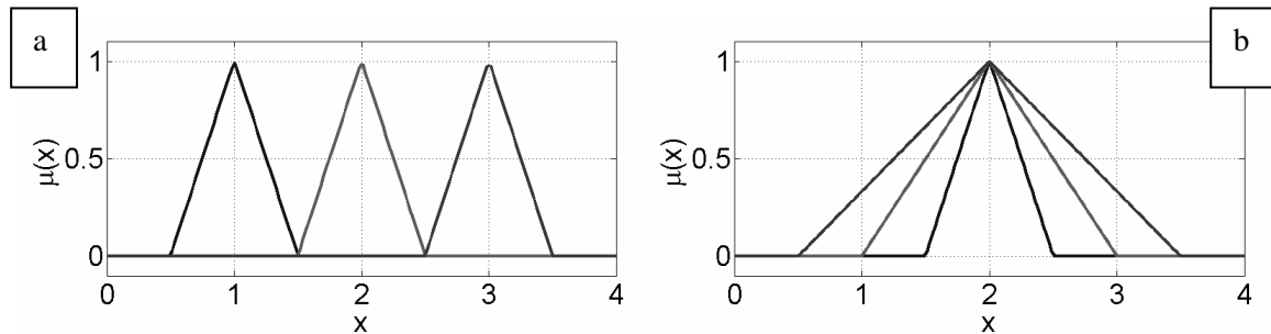
Fig. 6. Model input appartenance functions: a) the best of cases b) the worst of cases Rys. 6. Wzorcowe funkcje przynależności wejść: a) przypadek najlepszy, b) przypadek najgorszy
