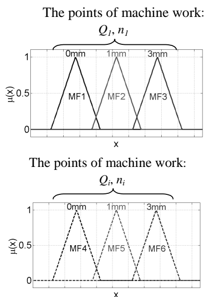
Fig. 10. System „II” of the rules construction system of fuzzy logic, MF1...6 – following appurtenance functions Rys. 10. System „II” budowy reguł systemu logiki rozmytej, MF1...6 – kolejne funkcje przynależności
