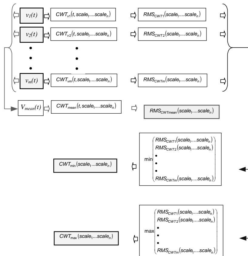
Fig. 3. The way of amplitude CWT change description Rys. 3. Sposób opisu charakteru zmian amplitudy CWT
