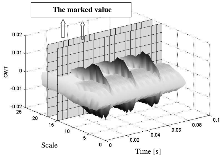
Fig. 3. The way of amplitude CWT change description Rys. 3. Sposób opisu charakteru zmian amplitudy CWT
