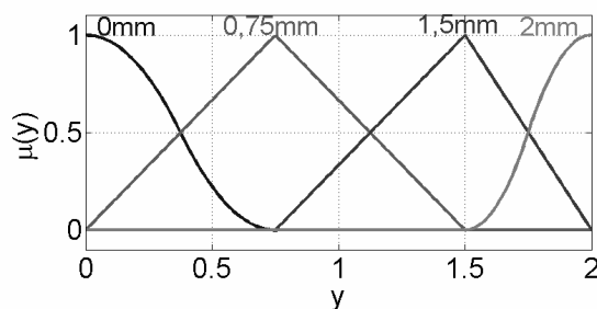
Fig. 8. Way number 2 of construction of the fuzzy outputs of the fuzzy logic system for a damage in the form of the chipping tip of the tooth Rys. 8. Sposób „2” budowy rozmytych wyjść systemu logiki rozmytej dla uszkodzenia w postaci wykruszenia wierzchołka zęba
