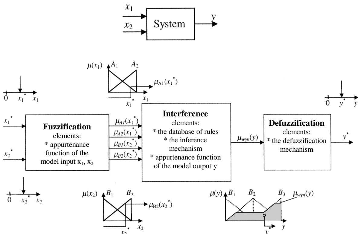
Fig. 1. The example structure of a fuzzy model Rys. 1. Przykładowa struktura modelu rozmytego
