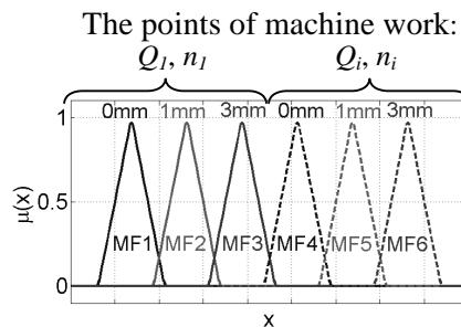
Fig. 9. System „I” of the rules construction system of fuzzy logic, MF1...6 – following appurtenance functions Rys. 9. System „I” budowy reguł systemu logiki rozmytej, MF1...6 – kolejne funkcje przynależności
